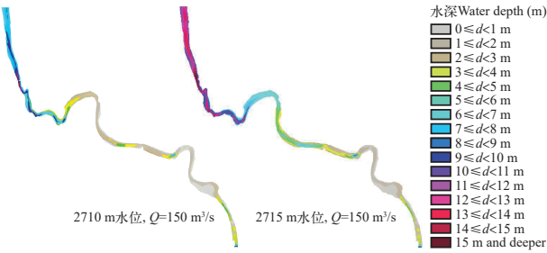
图 3 研究河段 2710 和 2715 m 水位典型流量下的水深分布
