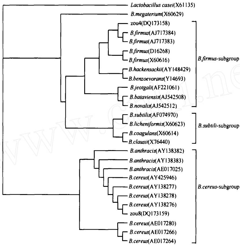
图3 菌株 zou4 和 zou8 的 16S rDNA 系统发育树 (括号内为序列登录号)
