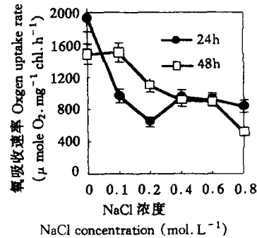
图3 NaCl对葛仙米光系统I(PSI)活性的影响.
