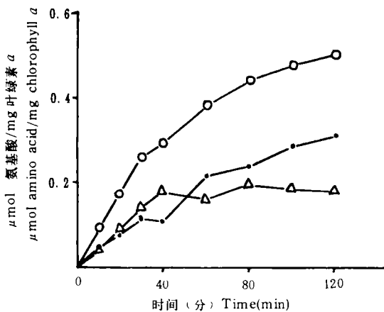
图 2 14 C 苯丙氨酸在微囊藻细胞中的代谢
