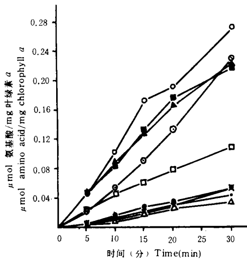
图 1 微囊藻对 14 C 标记氨基酸的吸收 ○: 丙氨酸; ⊙: 精氨酸; △: 天冬酰胺; ×: 天冬氨酸; ·: 谷氨酸; ■: 组氨酸; □: 亮氨酸; ▲: 赖氨酸; ●: 苯丙氨酸
