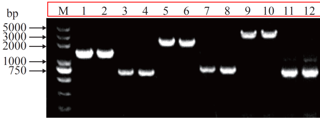
图 2 基因缺失株 \Delta amoA 、 \Delta amoE 、 \Delta amoF 菌落 PCR 鉴定
